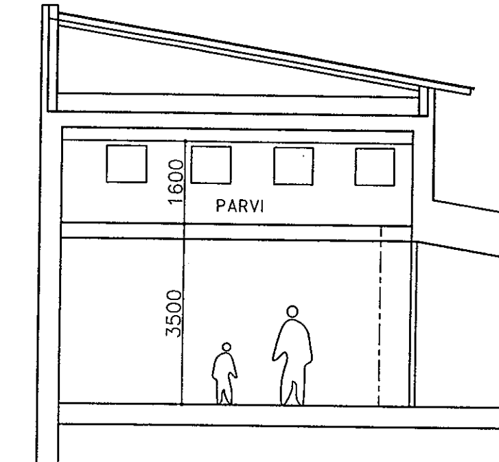
PARVEN LEIKKAUS
